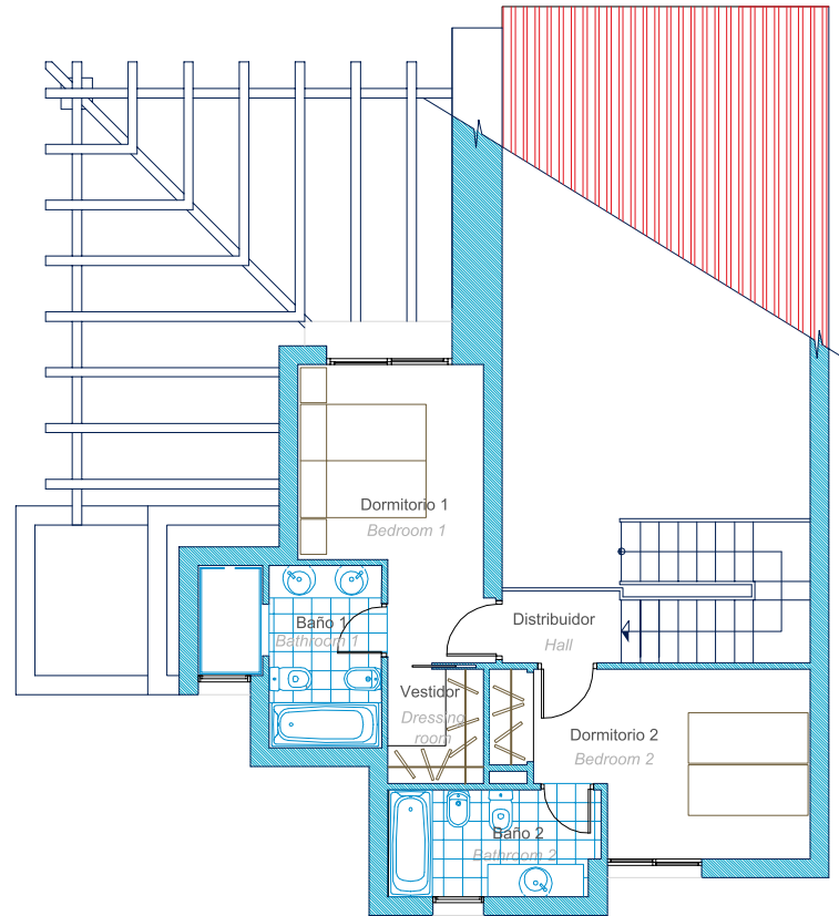
Planta Alta Top Floor
